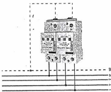
Układ połączeń ogranicznika ETITEC-WENT TNC-S-3F
