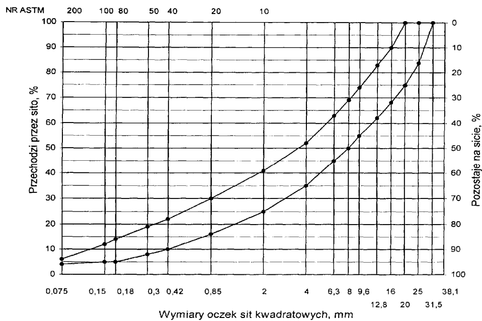
Rys. 6. Krzywe graniczne uziarnienia mieszanki mineralnej BA od 0 do 20 mm do warstwy wiążącej, wyrównawczej i wzmacniającej
