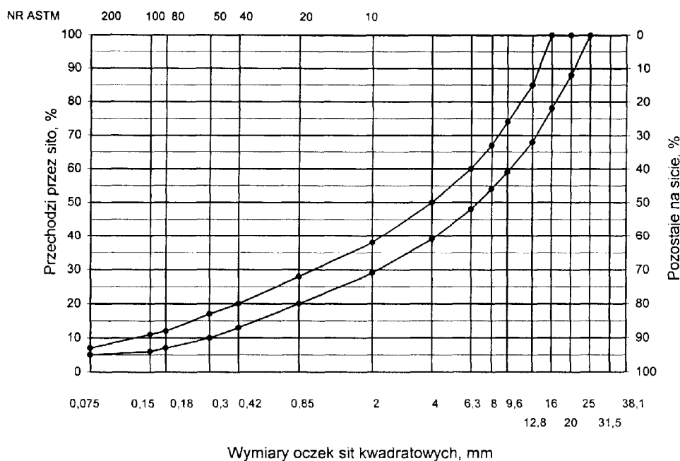
Rys. 1. Krzywe graniczne uziarnienia mieszanki mineralnej BA od 0 do 20 mm do warstwy ścieralnej
