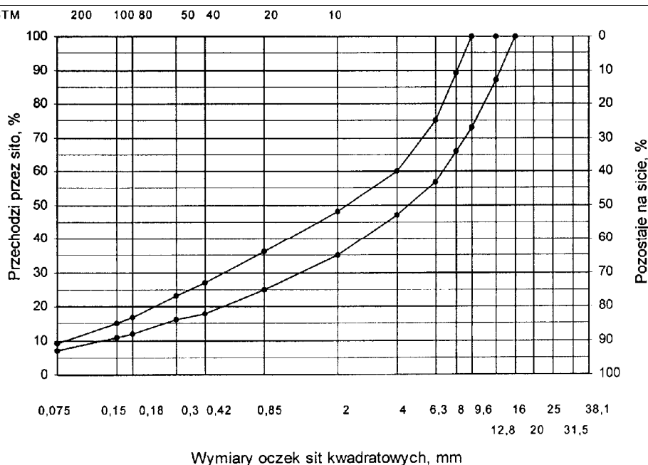
Rys. 4. Krzywe graniczne uziarnienia mieszanki mineralnej BA od 0 do 12,8 mm do warstwy ścieralnej
