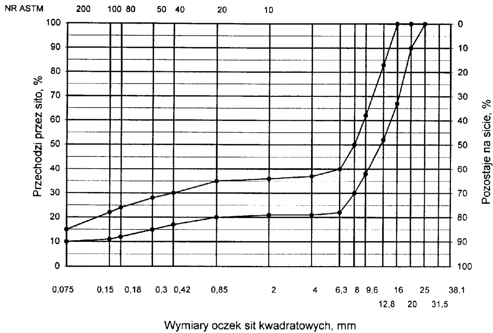
Rys. 2. Krzywe graniczne uziarnienia mieszanki mineralnej BA od 0 do 20 mm (mieszanka o nieciągłym uziarnieniu) do warstwy ścieralnej.
