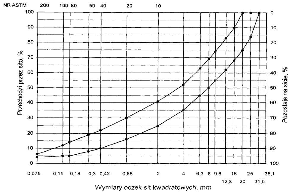
Rys. 5. Krzywe graniczne uziarnienia mieszanki mineralnej BA od 0 do 25 mm do warstwy wiążącej, wyrównawczej i wzmacniającej
