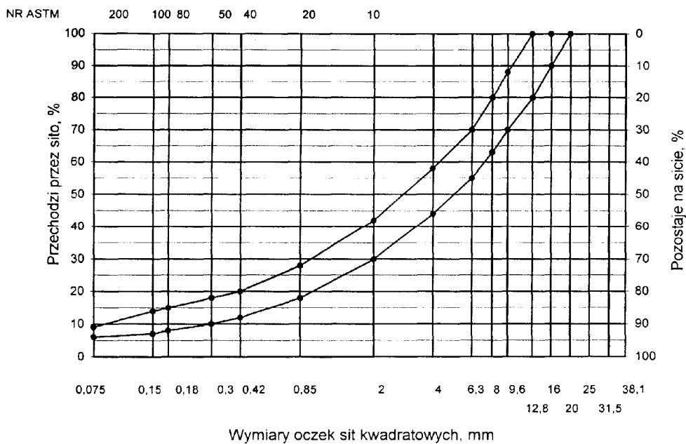
Rys. 3. Krzywe graniczne uziarnienia mieszanki mineralnej BA od 0 do 16 mm do warstwy ścieralnej
