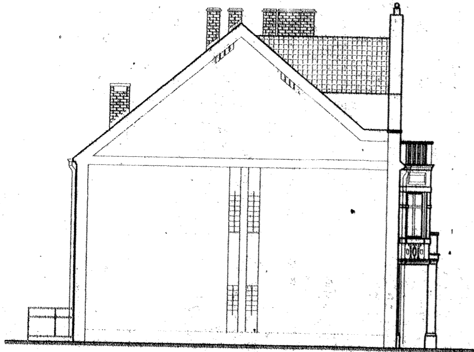
ELEWACJA BOCZNA
