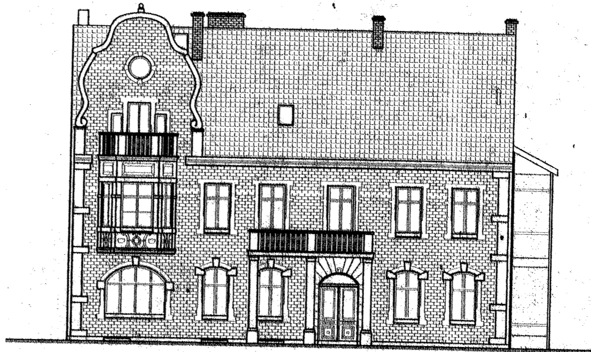
ELEWACJA FRONTOWA
