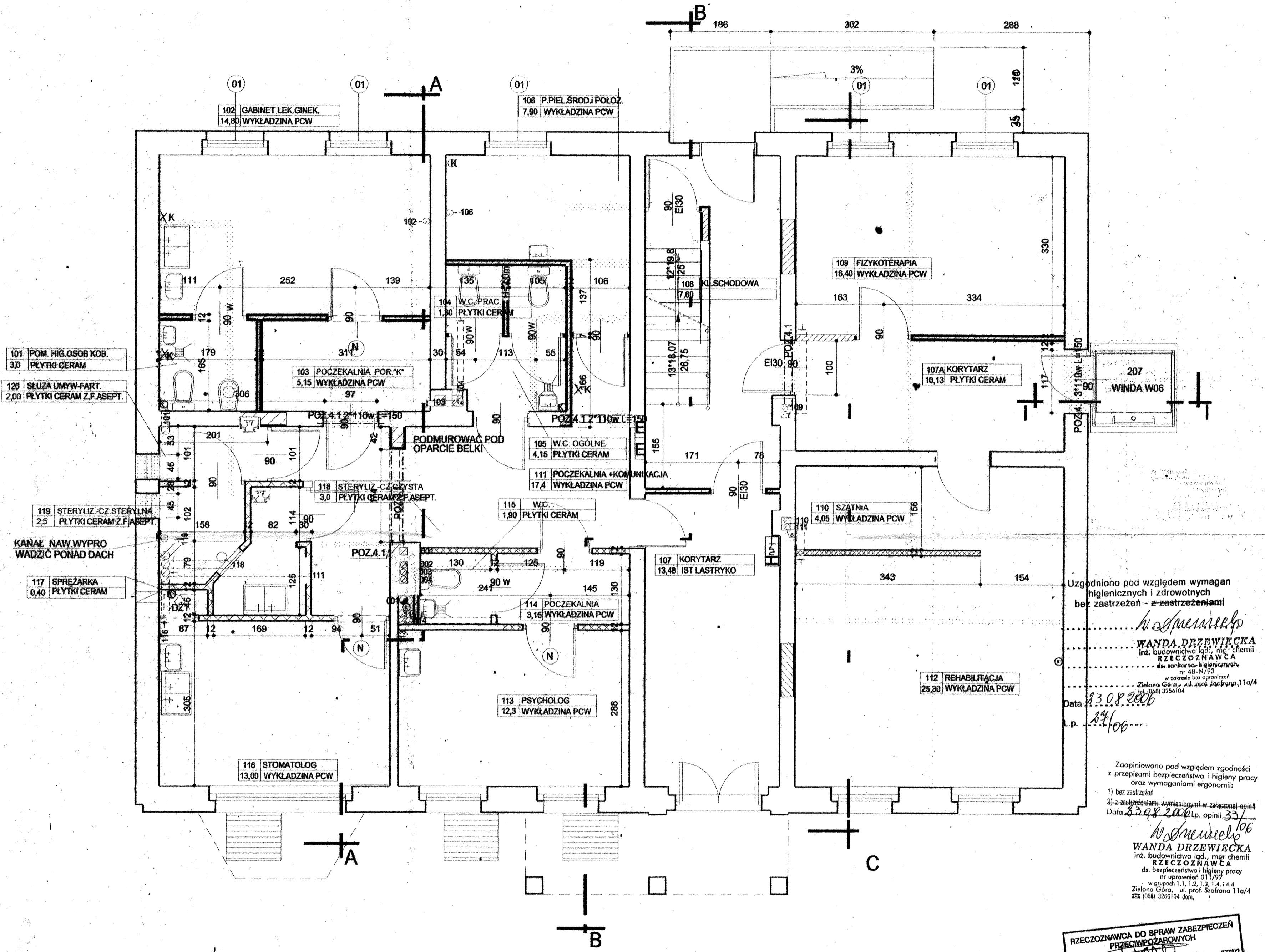
RZUT PARTERU
