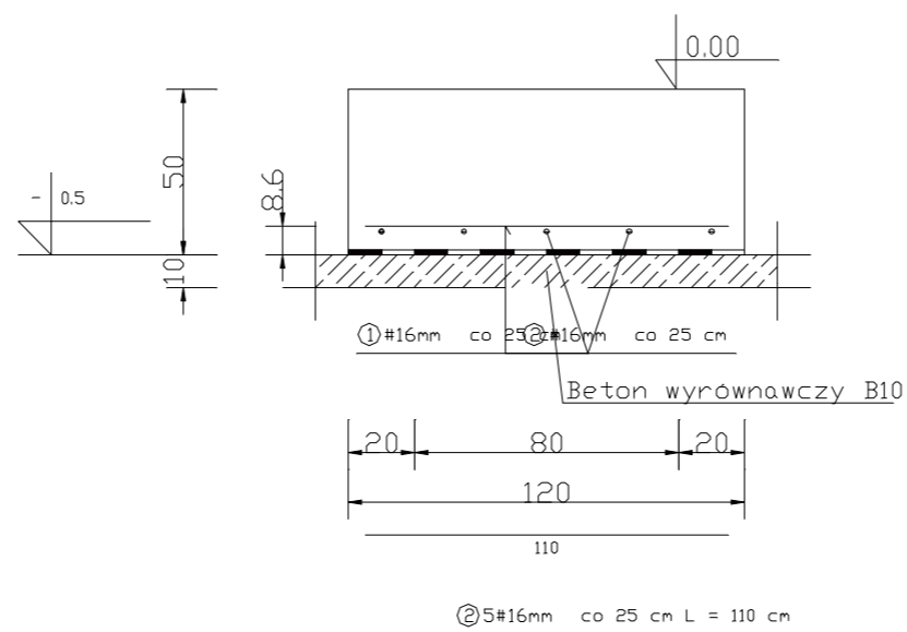
PRZEKRÓJ B-B
