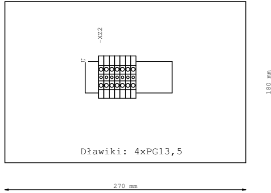
Skrzynka przyłączeniowa SP-Z2
