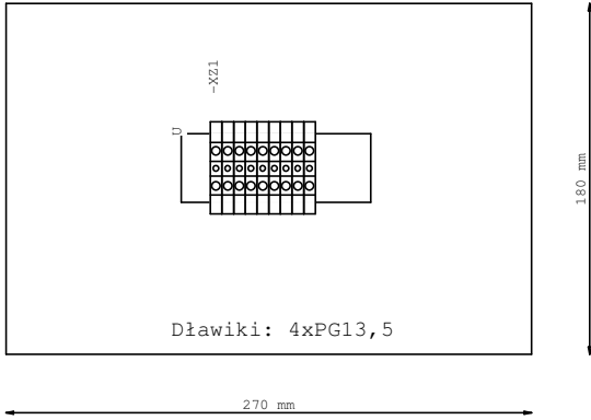
Skrzynka przyłączeniowa SP-Z1
