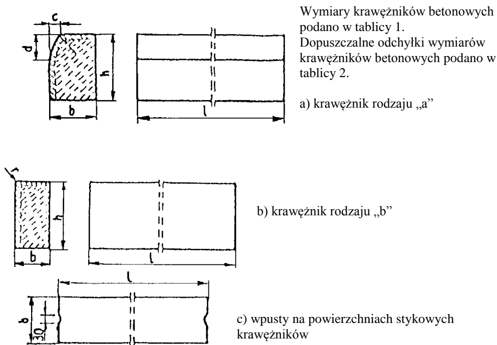
Rys. 1. Wymiarowanie krawężników
