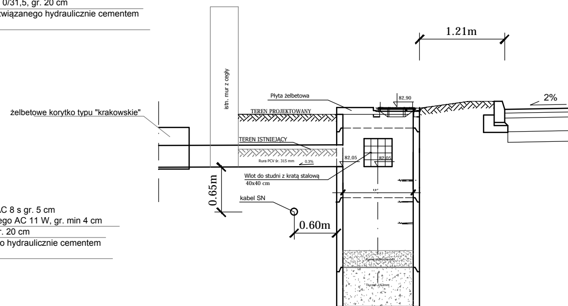
10. Przekrój normalny
