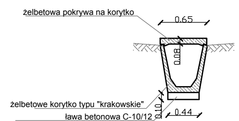
Przekrój rowu krytego B-B
