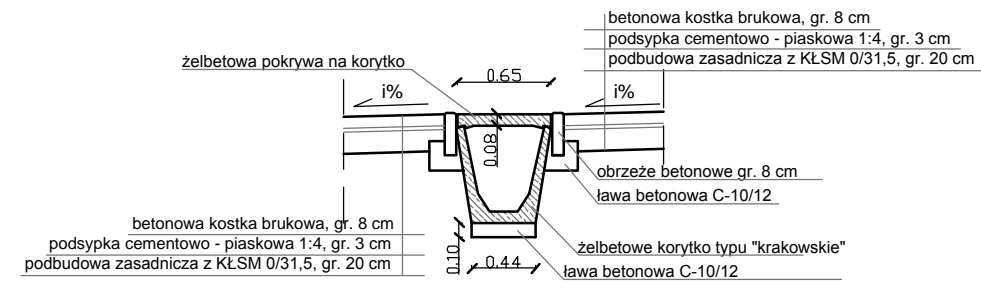
Przekrój rowu krytego A-A
