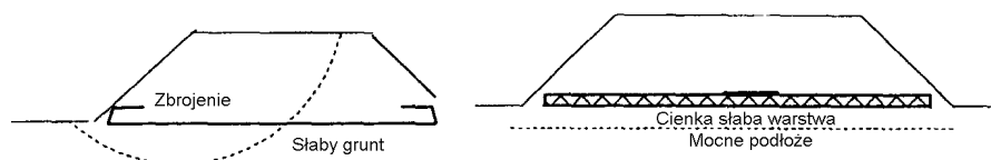
a - zbrojenie podstawy nasypu b - materac w podstawie nasypu
