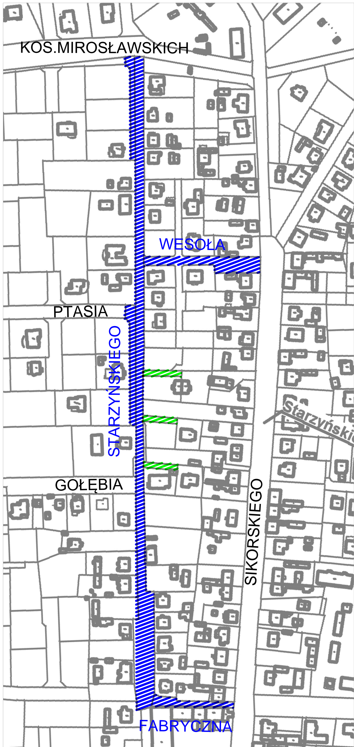
RYS.1 BUDOWA ULIC STARZYŃSKIEGO WESOŁEJ I FABRYCZNEJ W WITNICY ZE ZJAZDAMI
