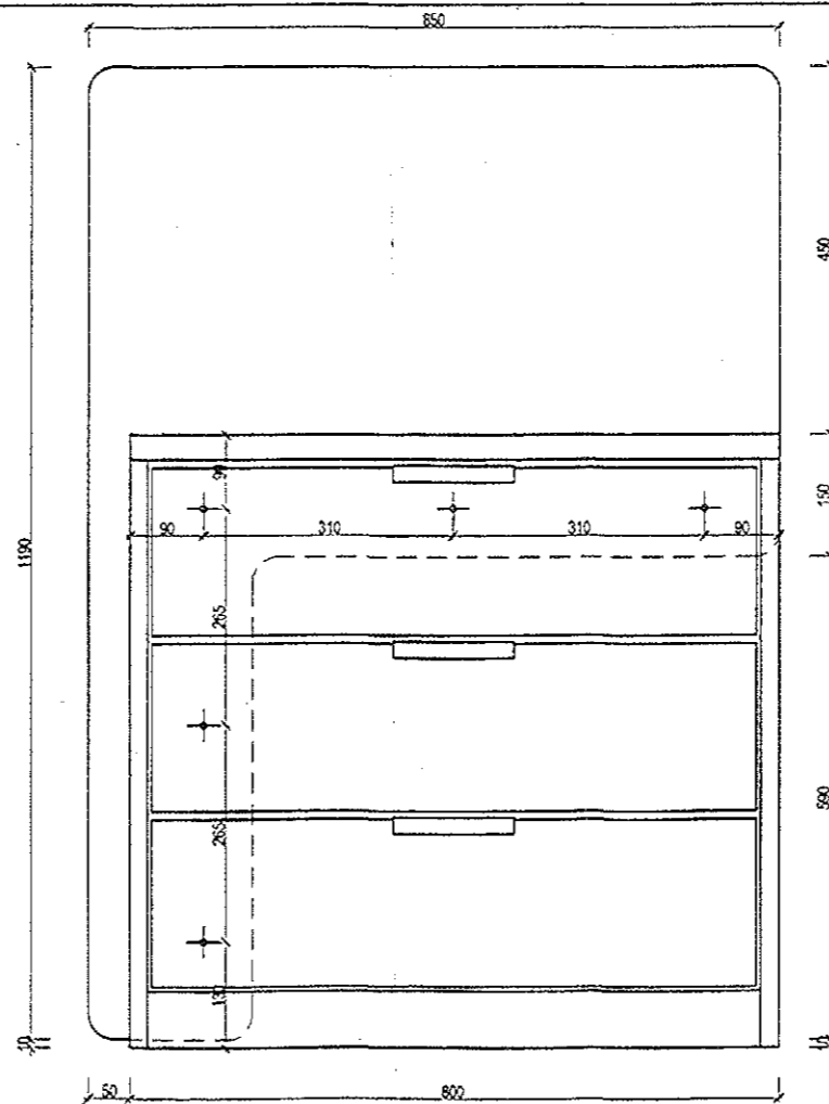
KŁAD FRONTOWY wersja podwójna_ skala 1:10
