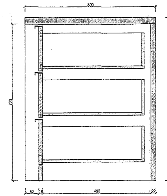
PRZEKRÓJ 1-1 wersja pojedyncza_skala 1:10
