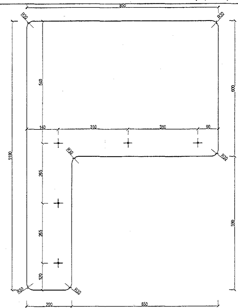
PLEKSI SZCZEGÓŁ_ skala 1:10
