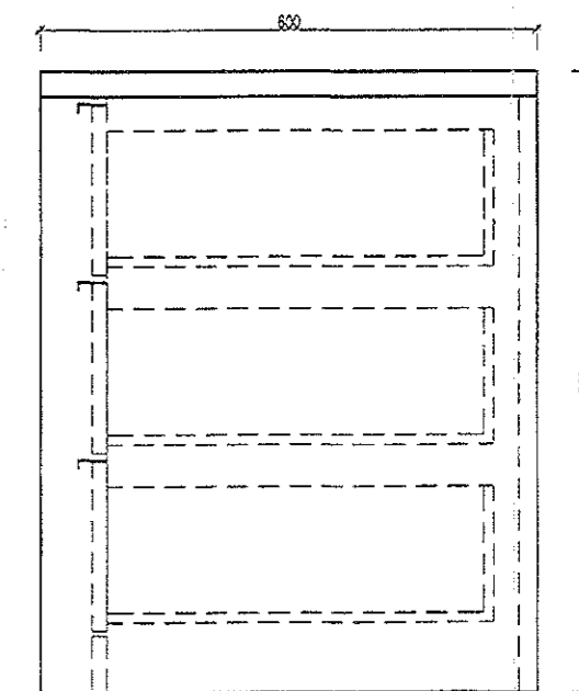
KŁAD BOCZNY wersja pojedyncza_skala 1:10
