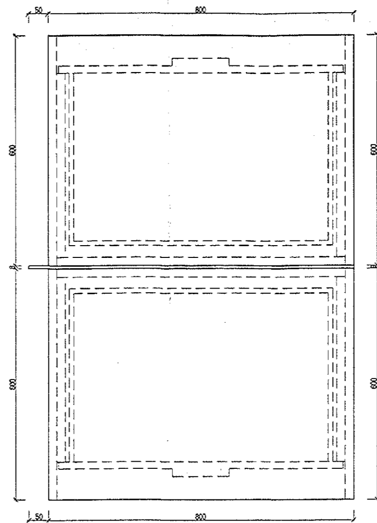
RZUT wersja podwójna_ skala 1:10
