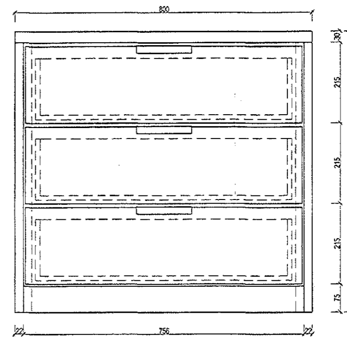
KŁAD FRONTOWY wersja pojedyncza_skala 1:10
