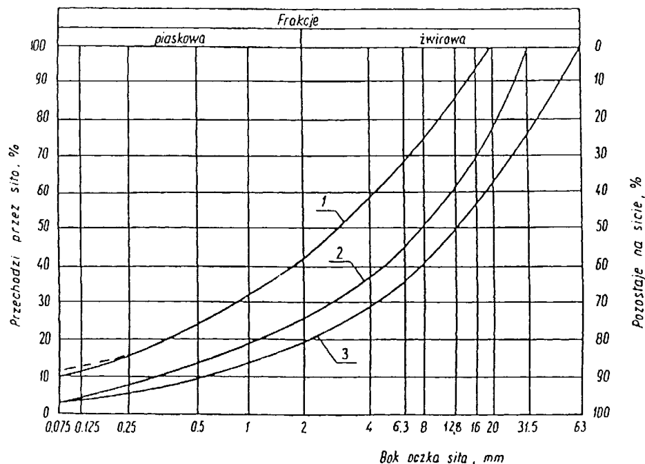
Rys. 1. Pole dobrego uziarnienia kruszyw przeznaczonych na podbudowy wykonywane metodą stabilizacji mechanicznej
