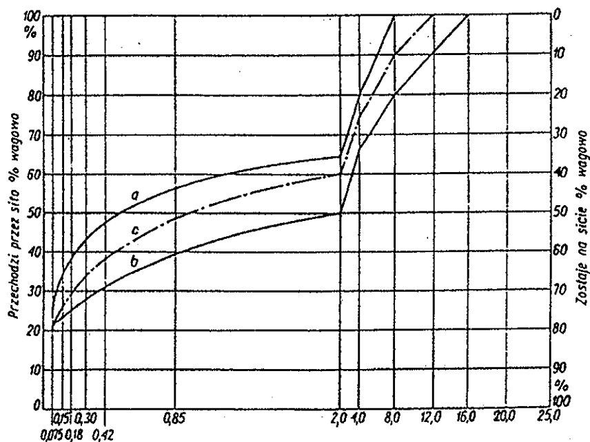
Rys. 2. Krzywe graniczne uziarnienia mieszanki mineralnej dla średnioziarnistej mieszanki asfaltu lanego: a, b - dla dróg międzymiastowych; b, c - dla dróg miejskich, mostów
