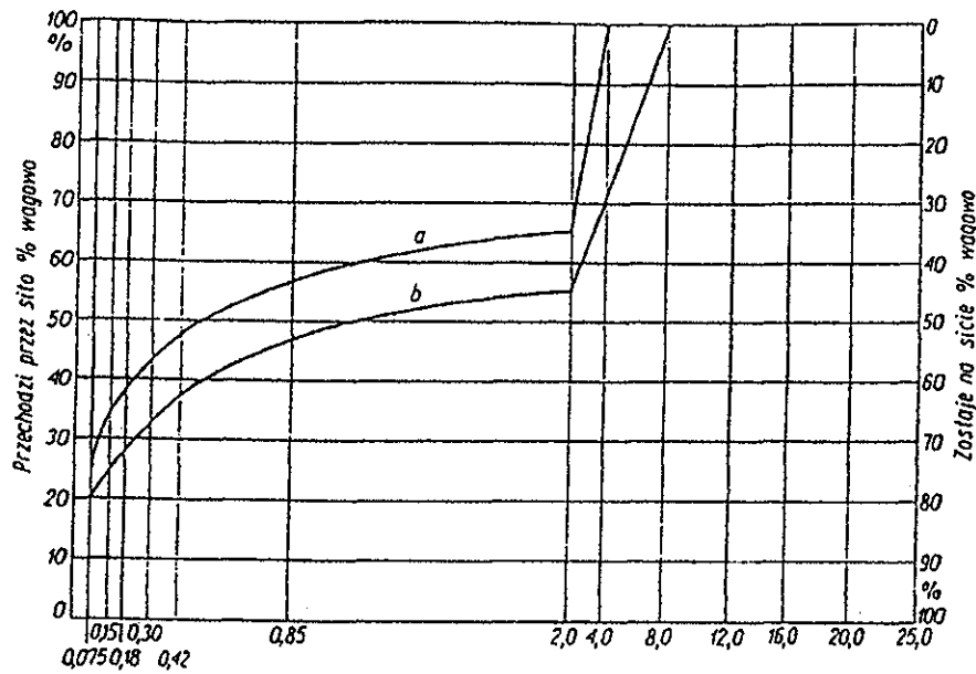
Rys. 3. Krzywe graniczne uziarnienia mieszanki mineralnej dla drobnoziarnistej mieszanki asfaltu lanego
