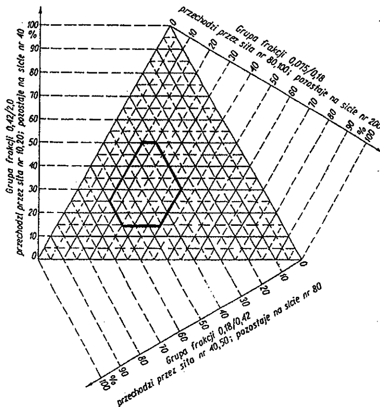
Rys. 4. Trójkąt Fereta
